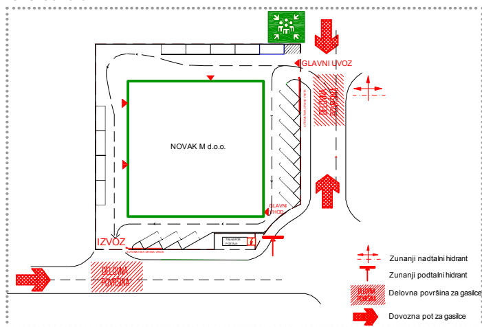
SITUACIJA OBJEKTA
